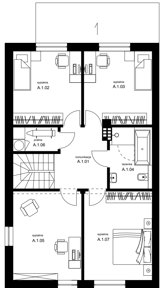
rzut piętra
