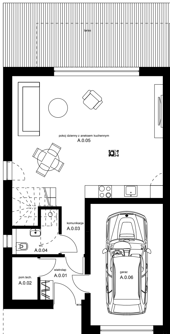
rzut parteru
