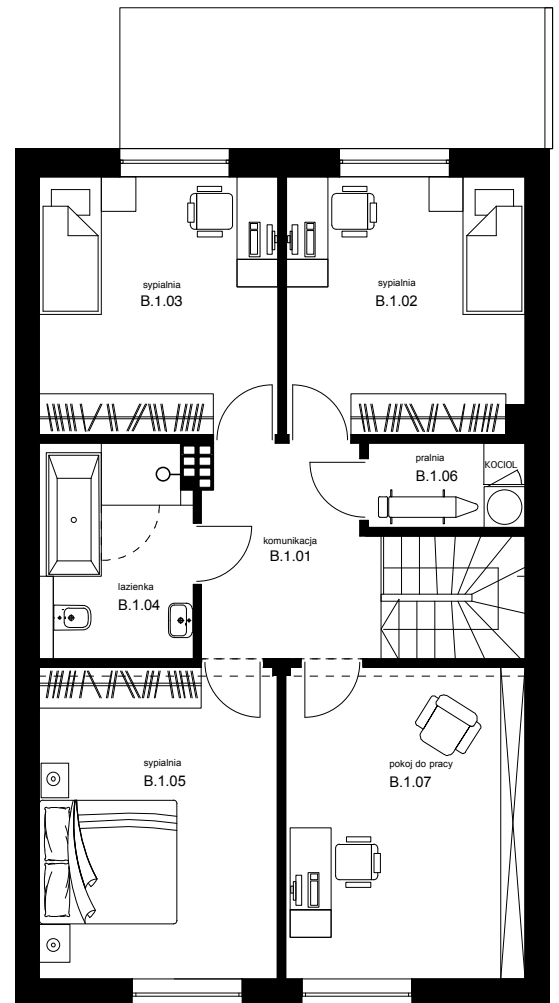
rzut piętra
