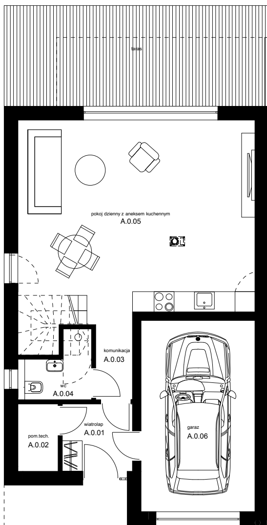
rzut parteru
