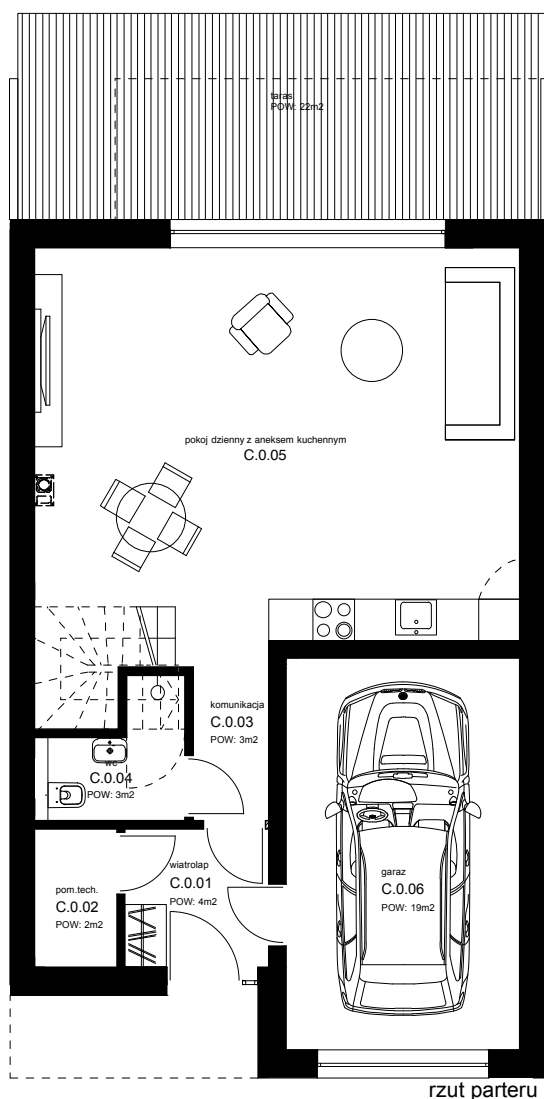
rzut parteru
